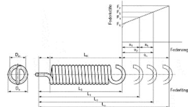
Sprężyny naciągowe
